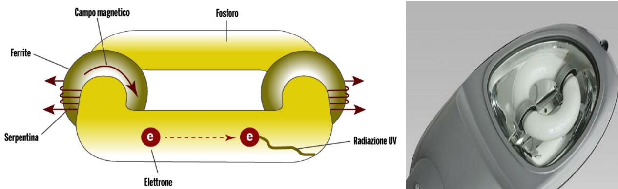
Figura 6.11 - lampada ad induzione
